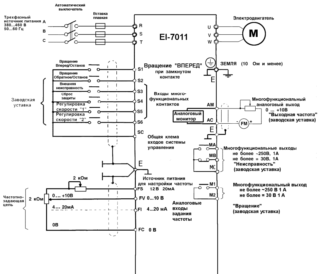
Рис. 9. Схема подсоединения.
